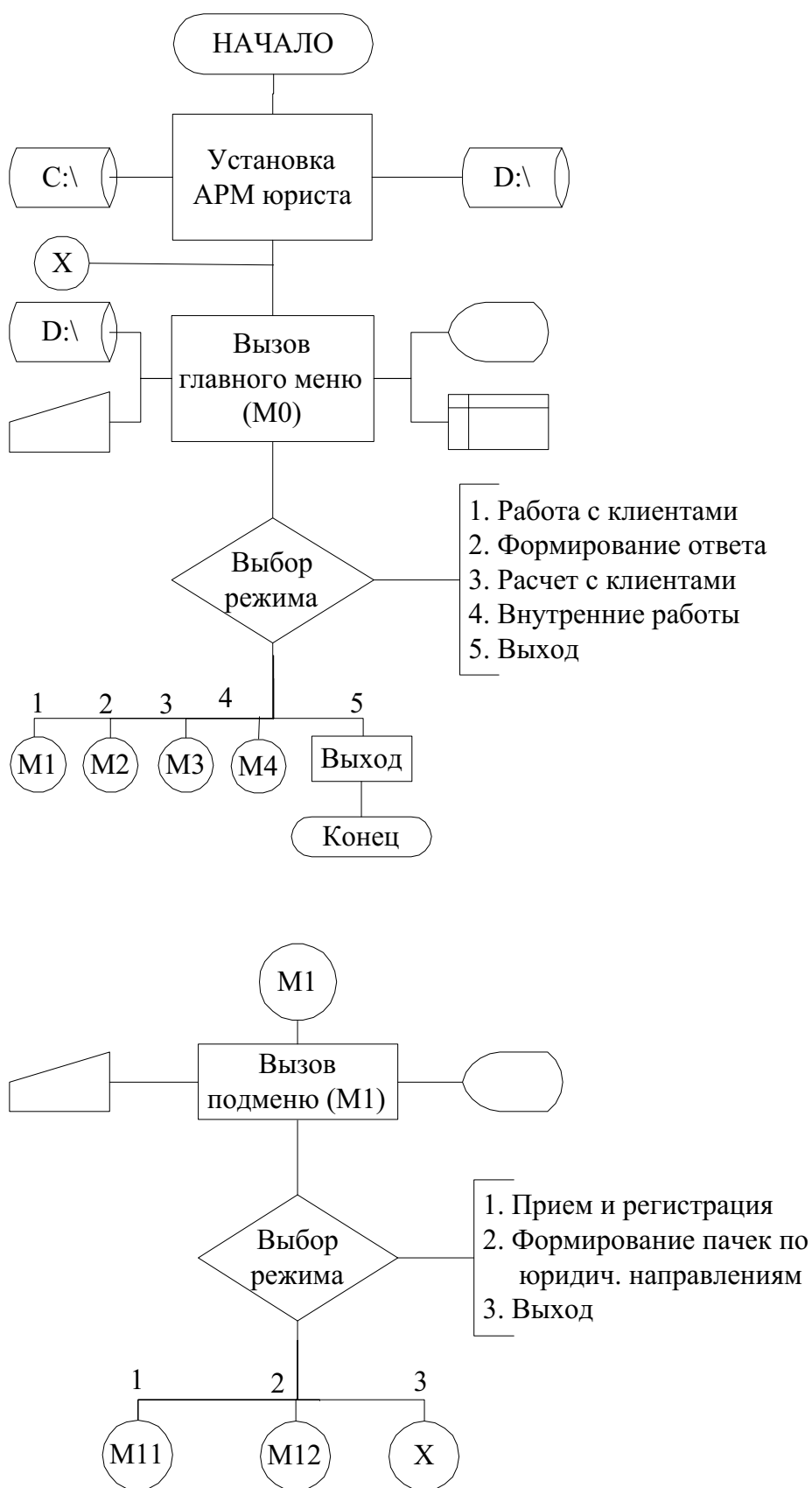
Рис 33. Схема работы системы АРМ юриста
