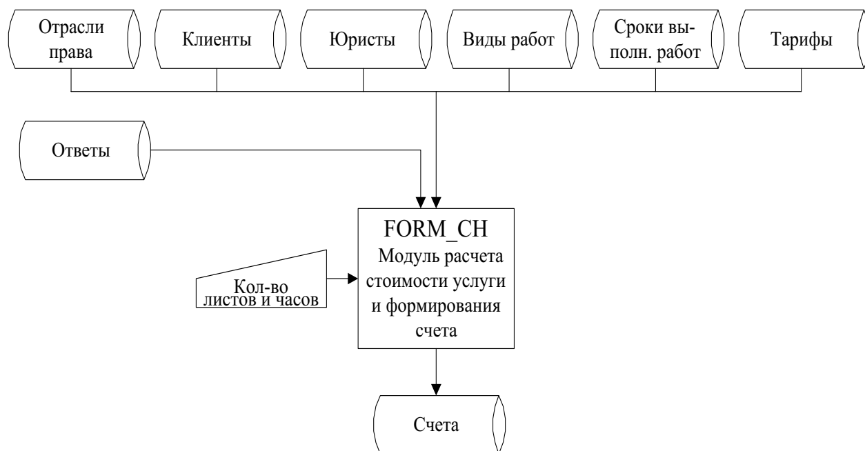
Рис.32. схема ресурсов модуля "Form_ch"
