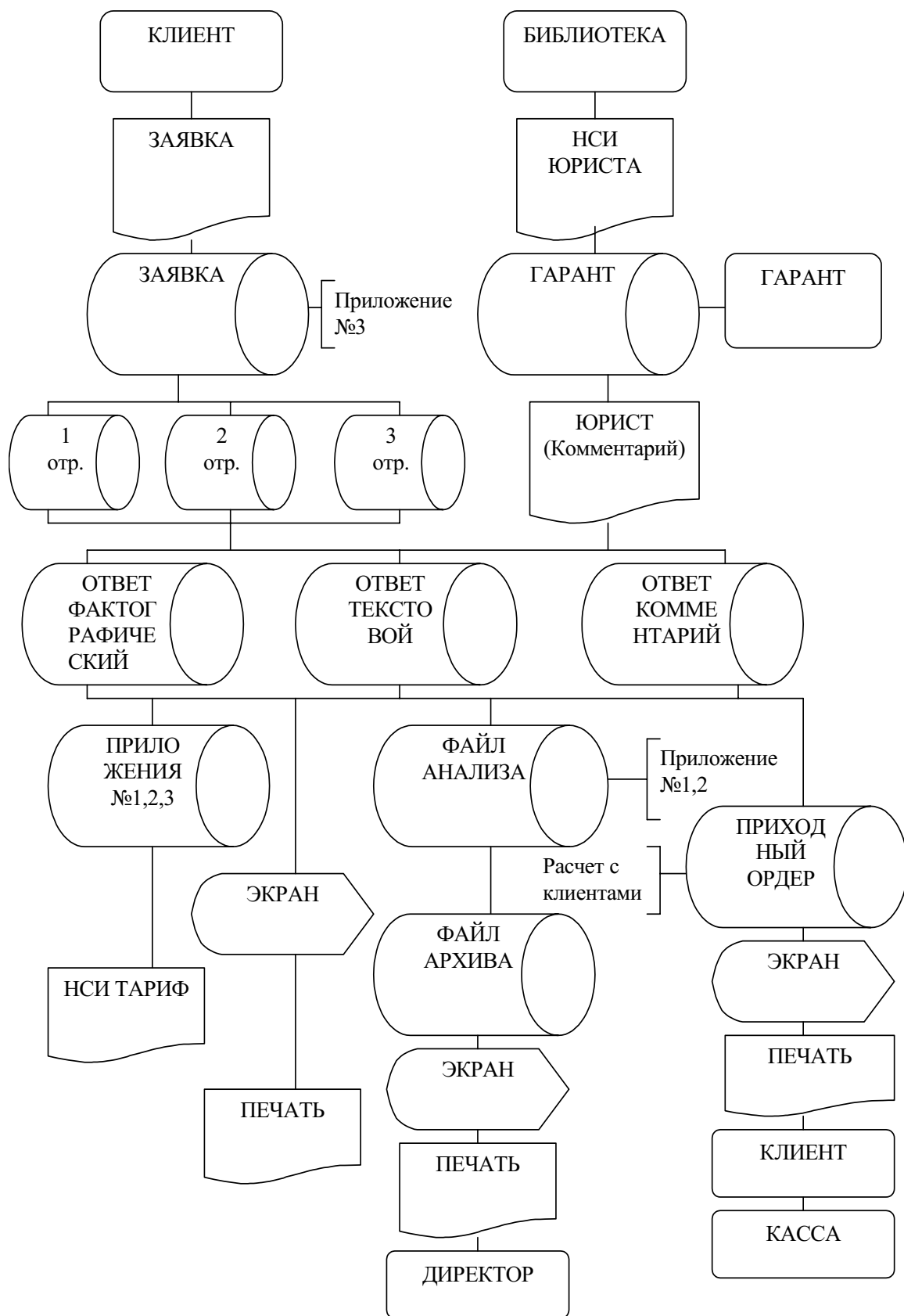
Рис. 27. Схема данных системы АРМ юриста по реализации консультативных юридических услуг
