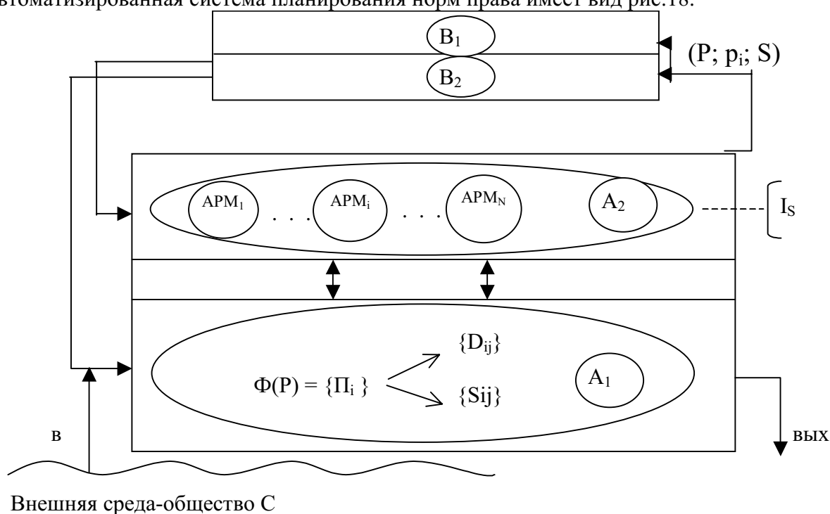
Рис. 18. Схема автоматизированной правовой системы
